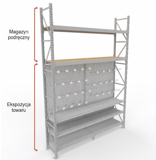
Przykładowy regał na wiertła
