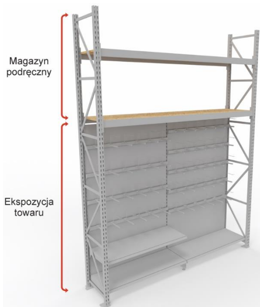
Przykładowy regał na tarcze i artykuły ściernie z tyłami gładkimi i wieszakami na belkę
