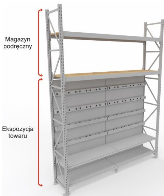
Przykładowy regał na baterie łazienkowe i kuchenne z tyłami gładkimi i wieszakami na belkę
