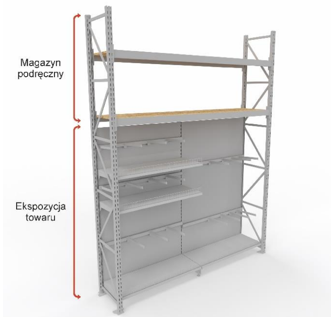
Przykładowy regał na akcesoria hydrauliczne z tyłami gładkimi i separatorami na belkę
